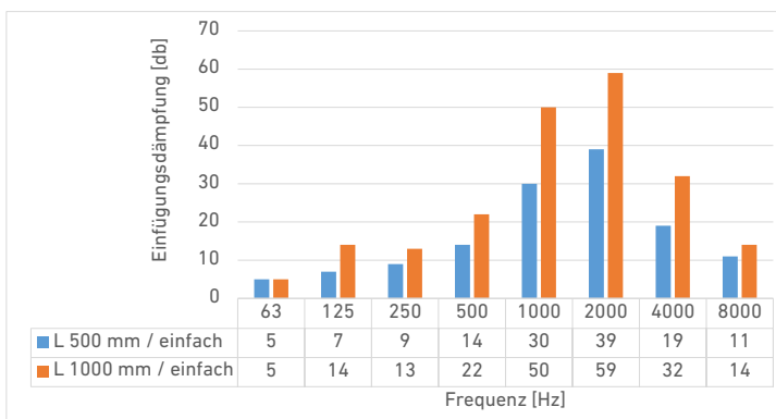
Einfügungsdämpfung
