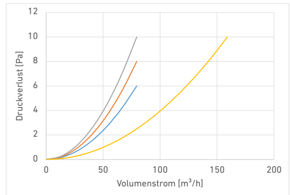
Druckverlust
