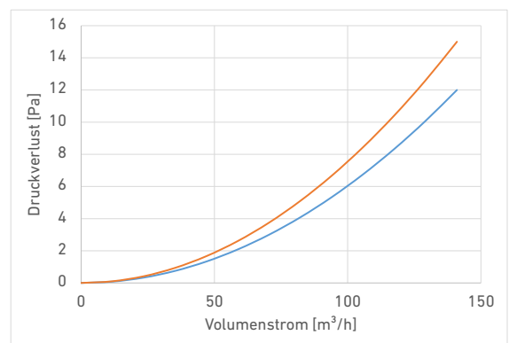
Druckverlust
