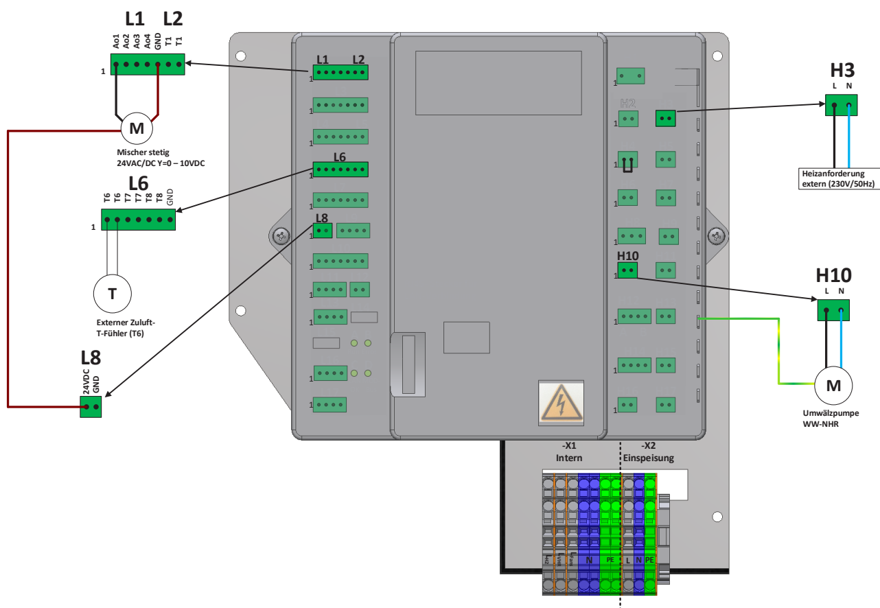
Abbildung: Anschlussbelegung für externes Warmwassernachheizregister
