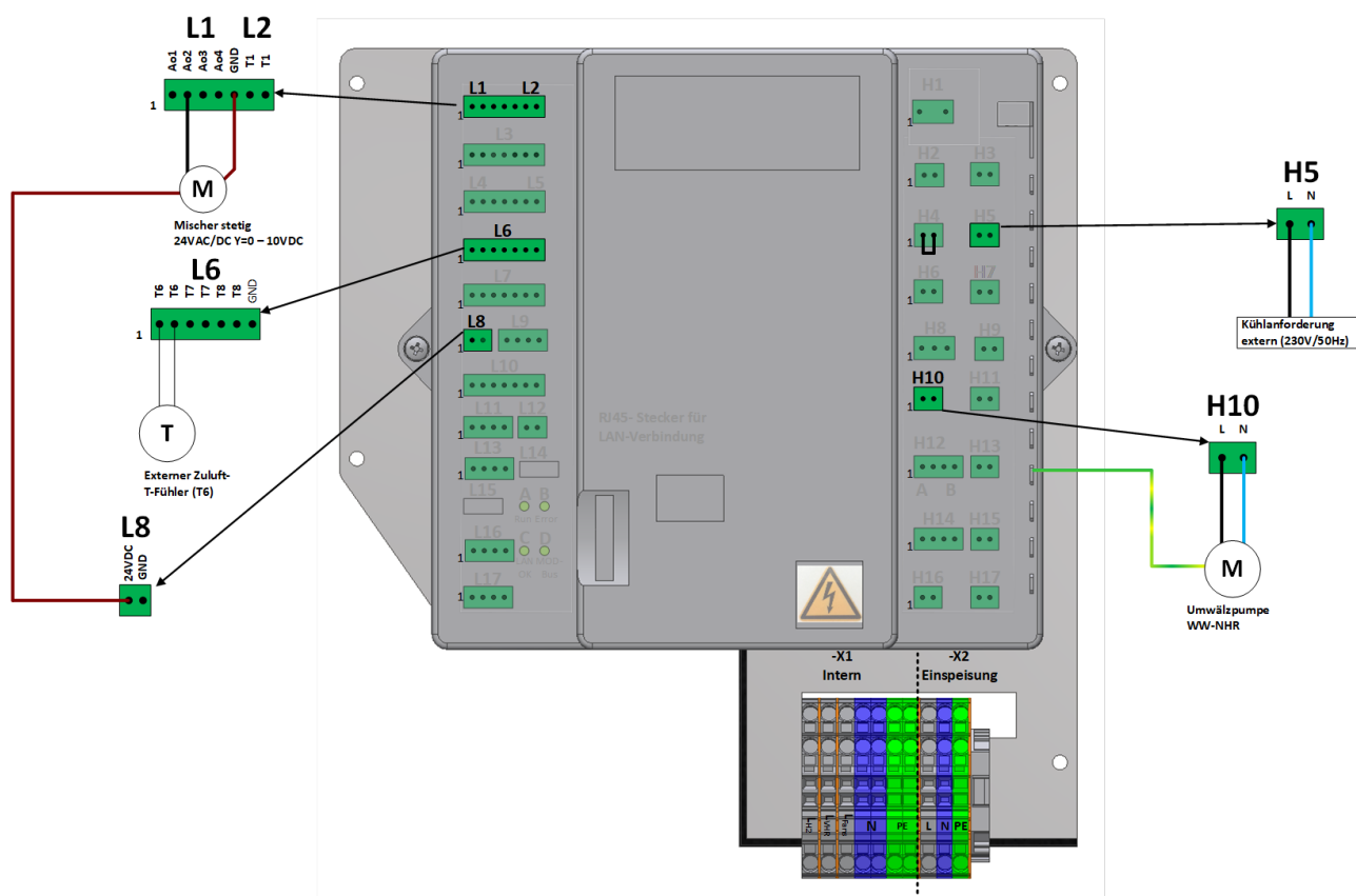
Abbildung: Anschlussbelegung für externes Kaltwasserkühlregister
