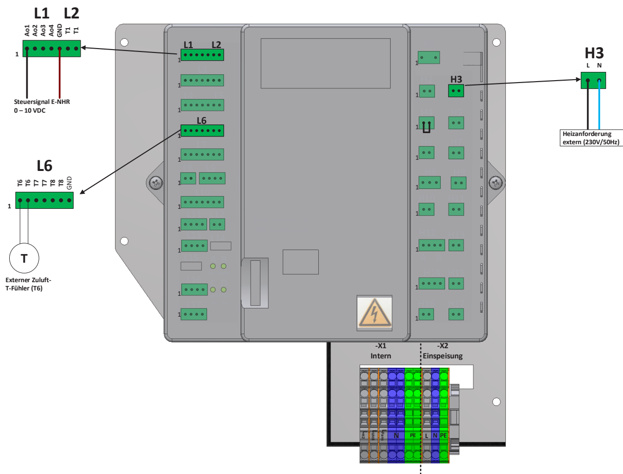
Abbildung: Anschlussbelegung für externes Elektronachheizregister
