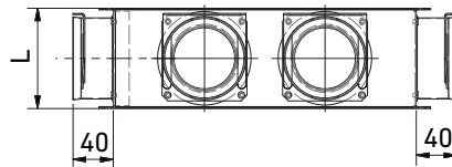
Ansicht Abluft
