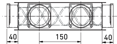
Ansicht Zuluft
