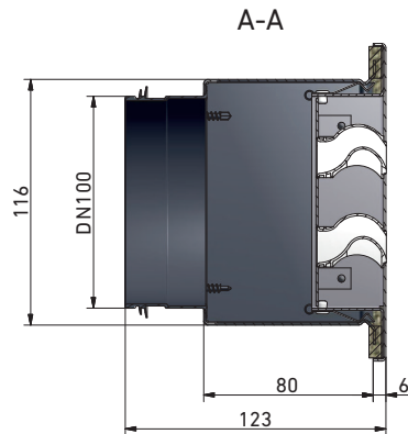
BKZ 100 mit Anschlusskasten
