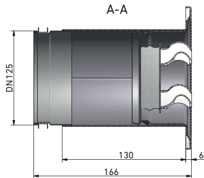
BKZ-R 125 mit Einbauhülse
