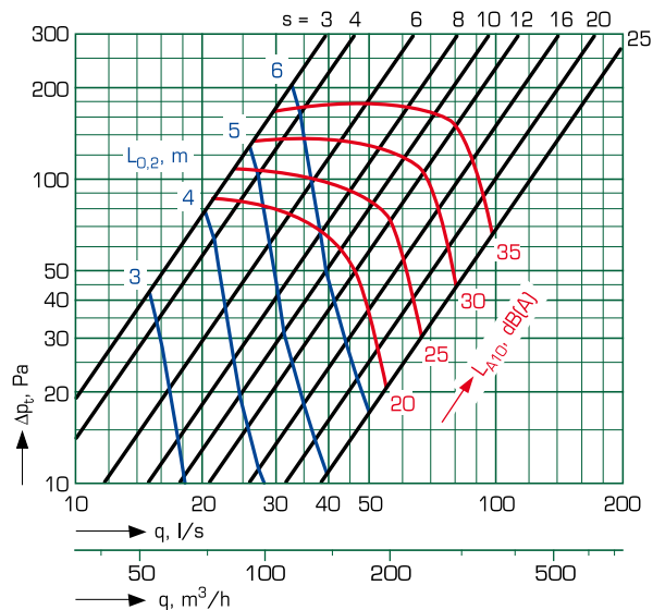
KTI-200
