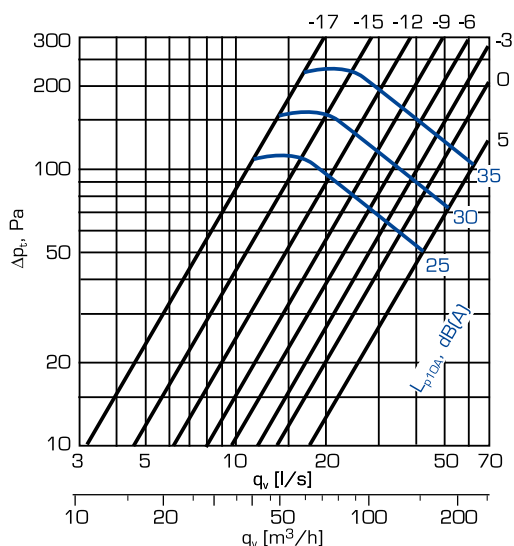
NK-160
