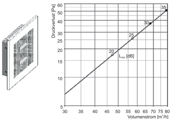
BKZ 100 ohne Drossel
