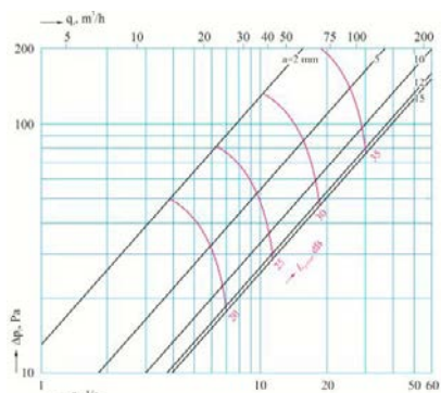
VST 080 mm
