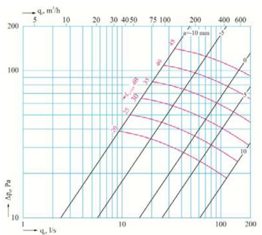
VEF 200 mm
