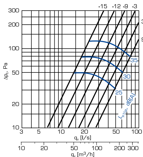
NK-200
