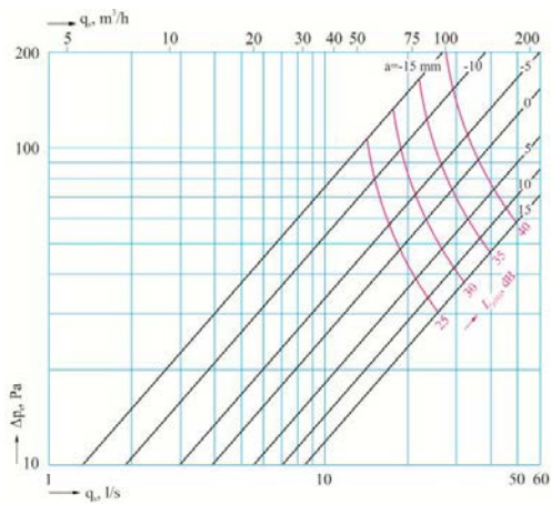
VEF 100 mm
