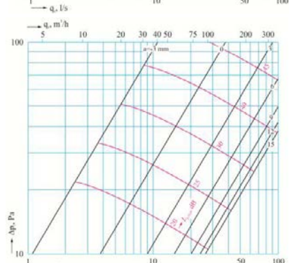
VST 160 mm innerer Schlitz geschlossen
