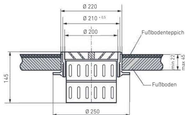
3. Einbauring 4. Schmutzfänger
