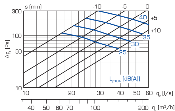
KSO-125
