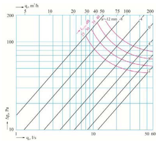
VEF 125 mm
