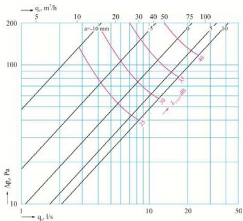
VEF 080 mm
