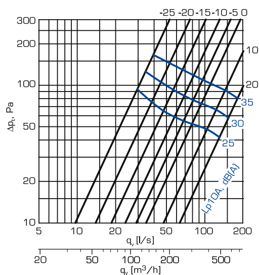
NK-200
