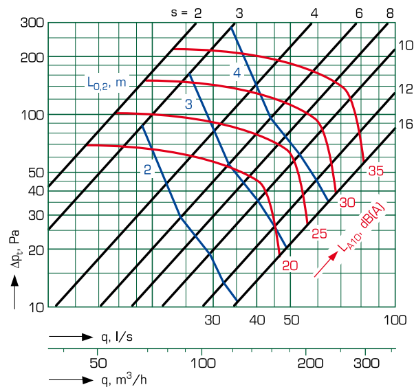
KTI-160
