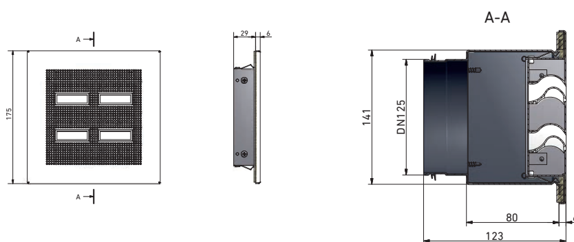
BKZ 125 (links) und BKZ 125 mit Anschlusskasten (ganz rechts)
