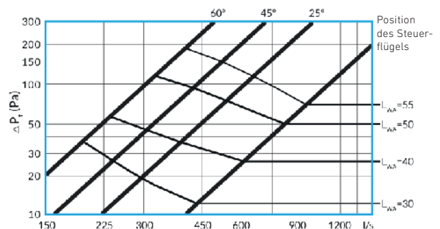
Sava-315
