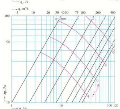
VST 200 mm innerer Schlitz geschlossen
