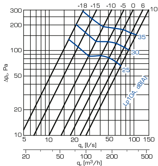
NK-160
