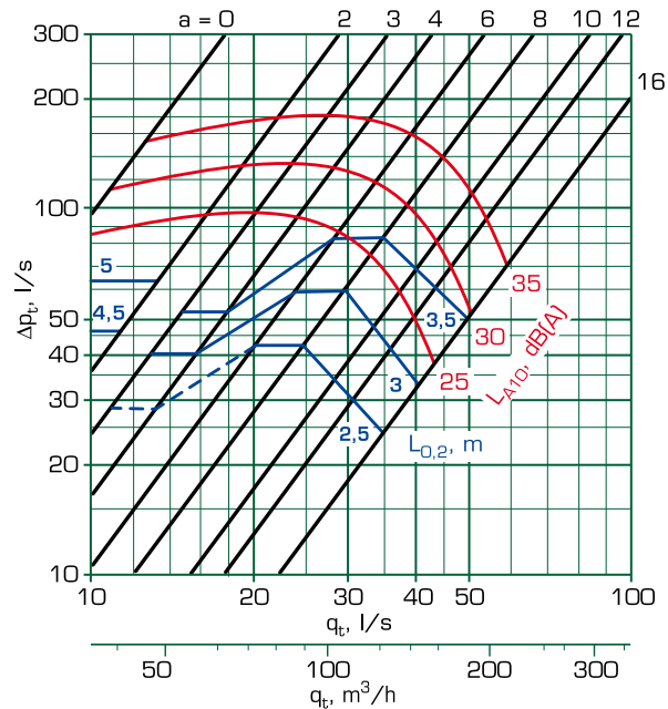
STI-160
