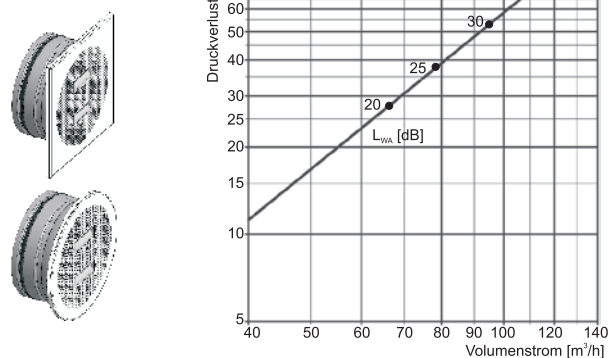
BKZ-R 125 ohne Drossel
