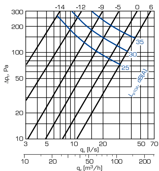
NK-150
