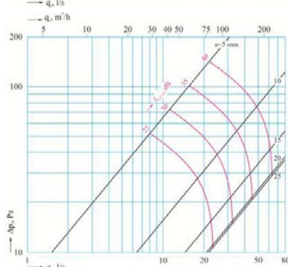
VST 100 mm
