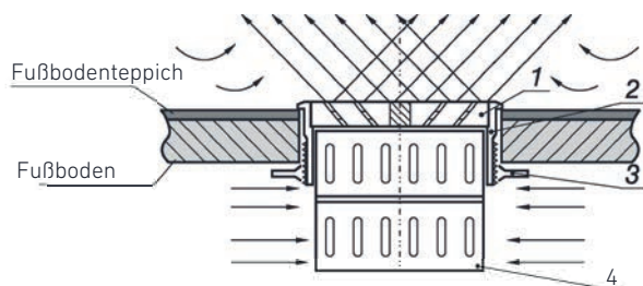
1. Luftauslass 2. Einbauflansch
