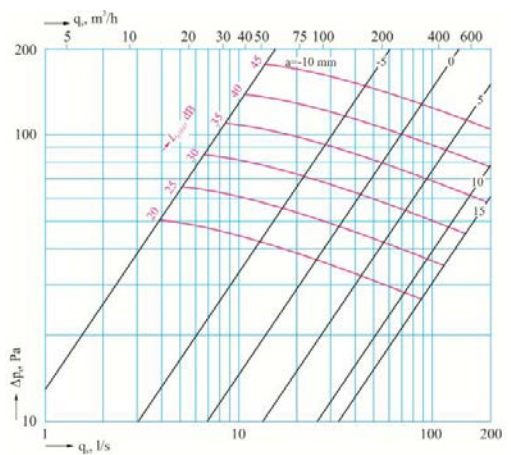
VEF 160 mm
