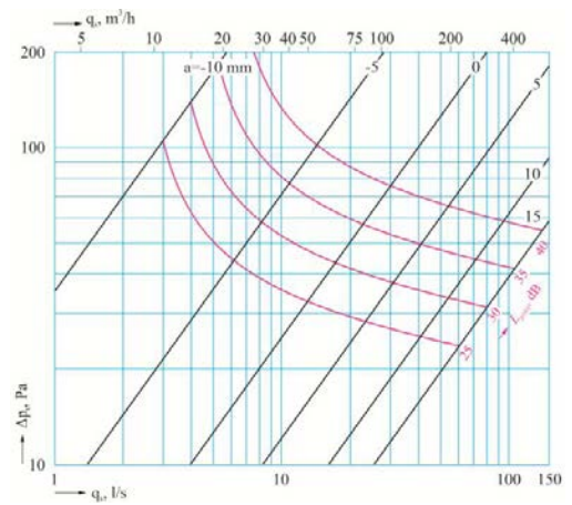
VEF 150 mm
