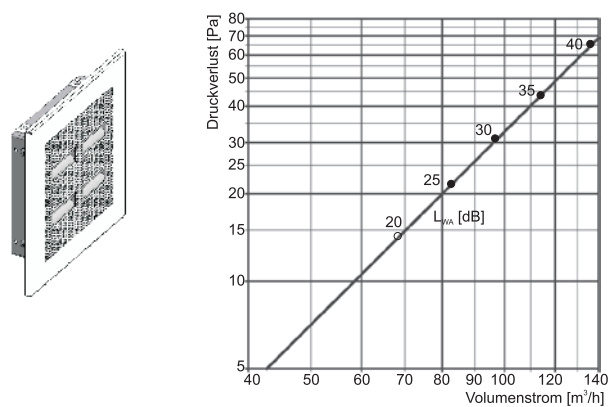
BKZ 125 ohne Drossel
