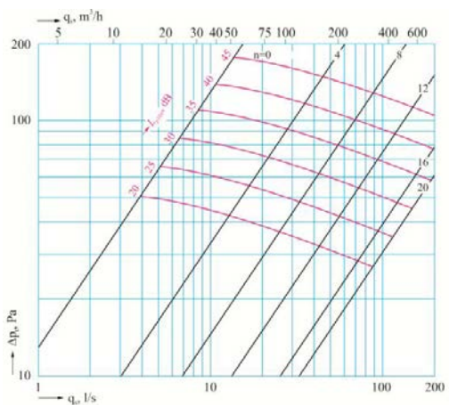
VEF 160 mm
