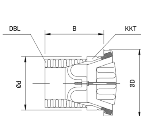
Abluftventil
