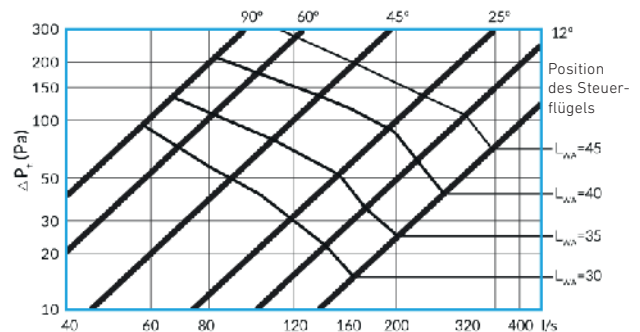
Sava-200
