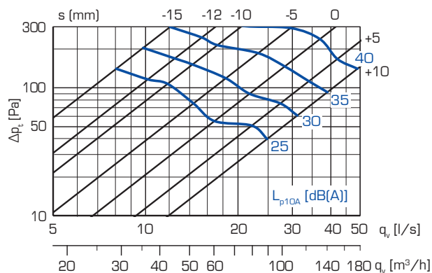
KSO-100
