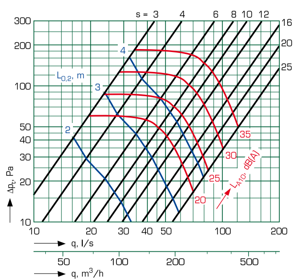
KTI-200
