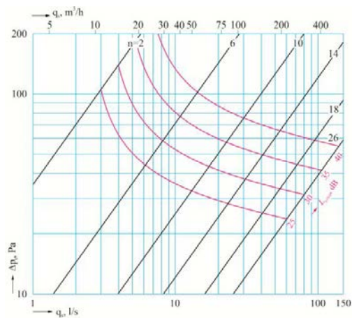
VEF 150 mm
