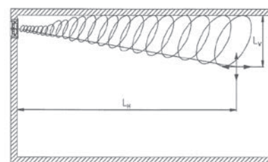
Abb. 1 Einsatzbedingungen und Einsatzbereiche für die verschiedenen Bautypen und Baugrößen. *Düsen mit 30° Ausblaswinkel, bei Düsen mit 45° erhöht sich die horizontale Wurfweite um 15 %
