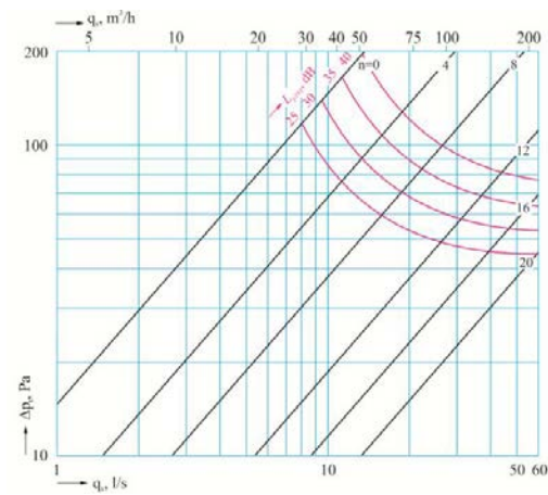
VEF 125 mm
