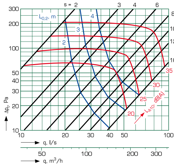
KTI-160
