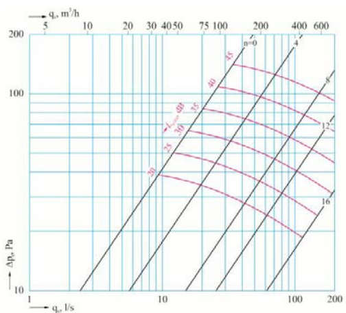
VEF 200 mm
