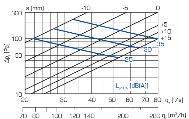
KSOV-160 + DBL-160
