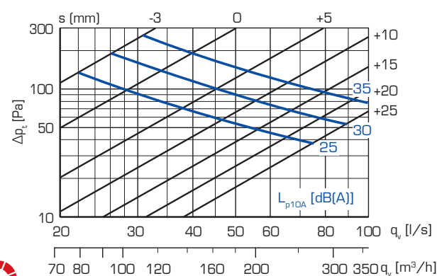
KSOV-200 + DBL-200
