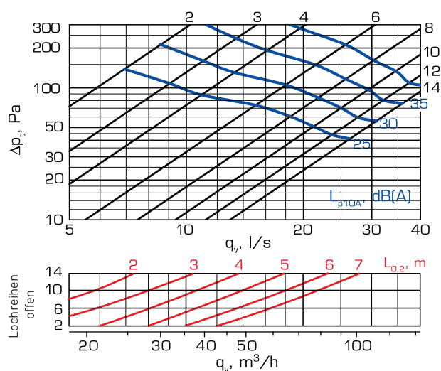
STQA-125
