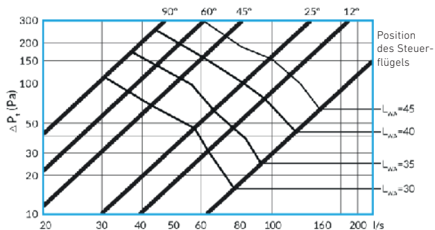
Sava-160
