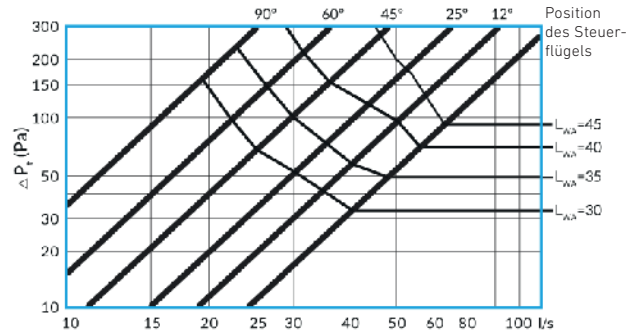
Sava-200
