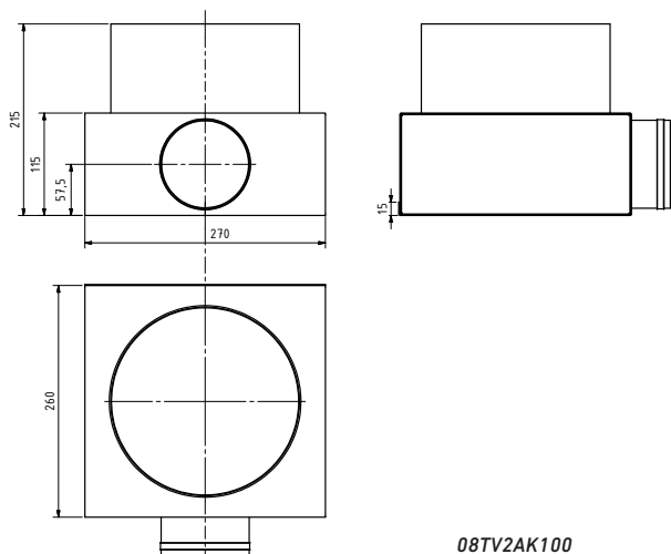
08TV2AK100
