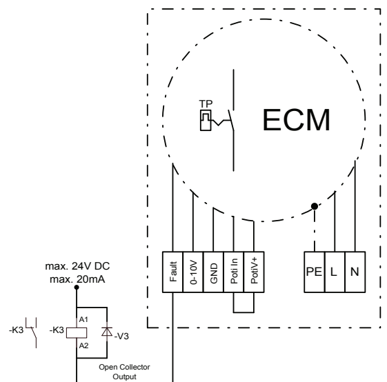
Relais mit Alarmausgang geschaltet
