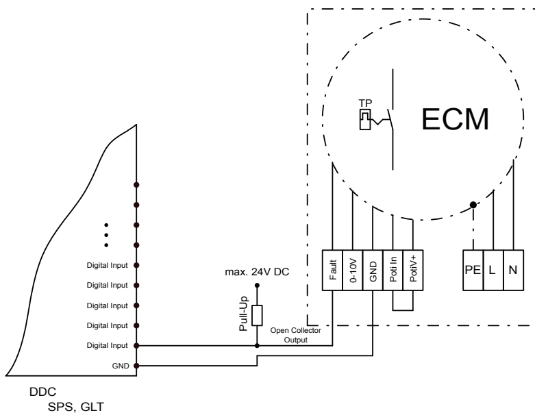
Alarmausgang auf Stererung aufgelegt
