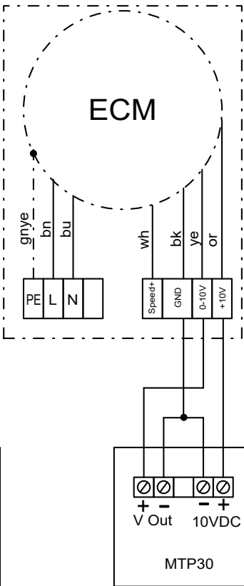
Anschluss Potentiometer MTP30
