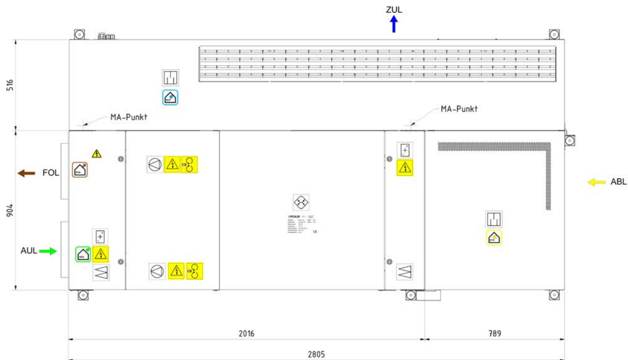
Linke Geräteausführung
