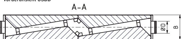
Draufsicht (Schnittdarstellung) USDD
