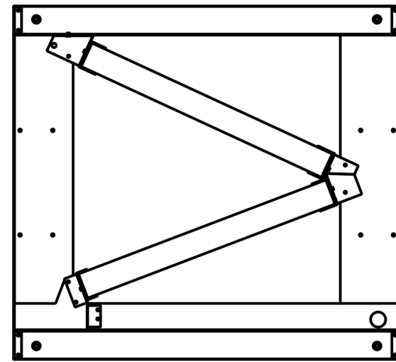
F-F ( 1 : 10 )
