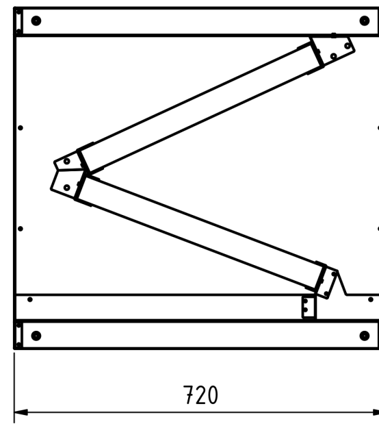
E-E ( 1 : 10 )
