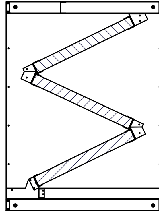
F-F ( 1 : 10 )
