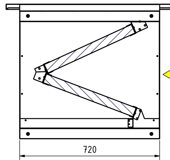
E-E ( 1 : 10 )
