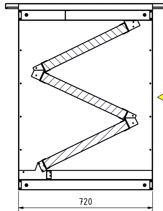
F-F ( 1 : 10 )
