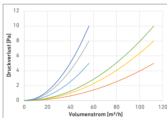
Druckverlust
