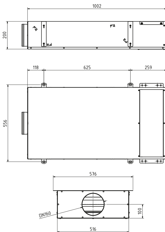
08USDABK160
