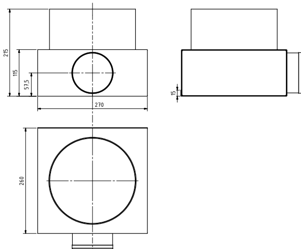
08TV2AKD100
