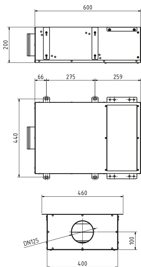
08USDABK125
