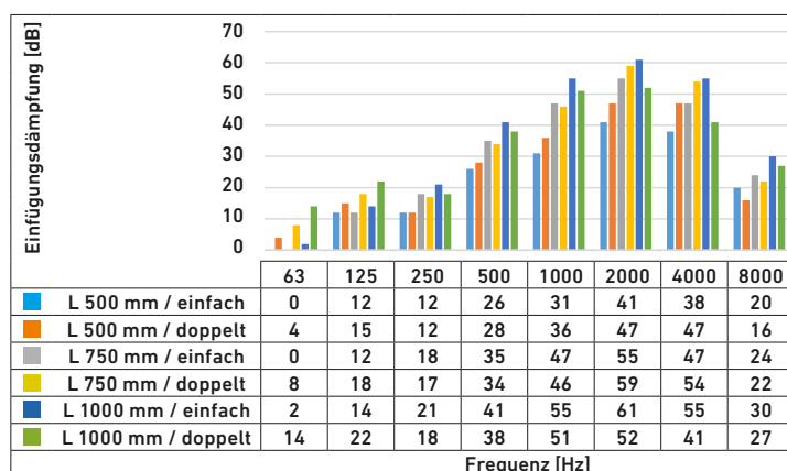
Einfügungsdämpfung
