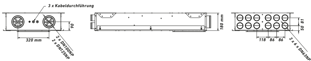
AUSFÜHRUNG SPIRO/SPIRO
