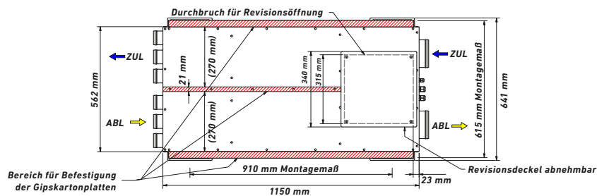
AUSFÜHRUNG SPIRO/KOMFLEX
