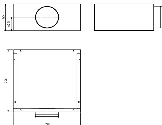
08TV2AKD100
