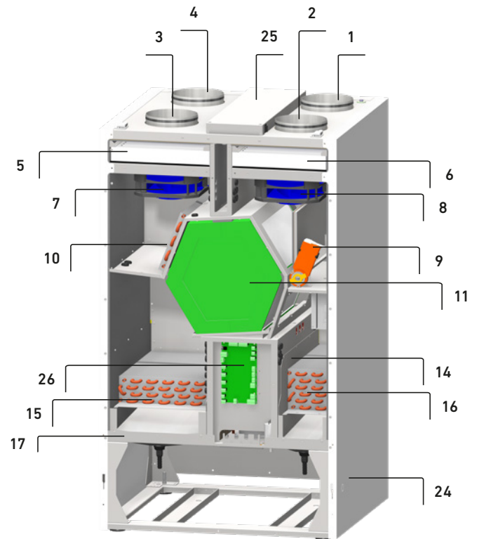
PKOM 4 A/AK TREND (RECHTE AUSFÜHRUNG)
