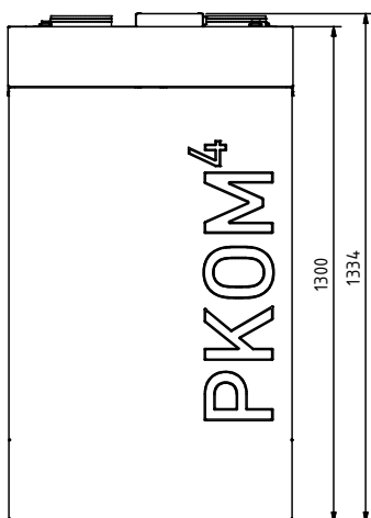
Abbildung: PKOM 4 A/AK trend (rechte Ausführung)
