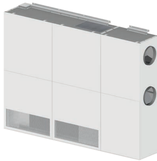
STANDGERÄT LG 1000 SKS mit Schalldämpfern in der ZUL/ABL und SD-Modul in der FOL/AUL
