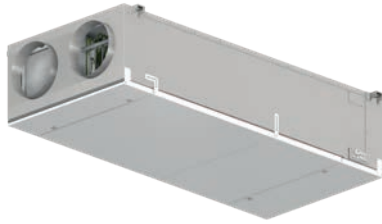
DECKENGERÄT LG 1000 SKDE mit SD-Modul, seitlich und unten ausblasend
