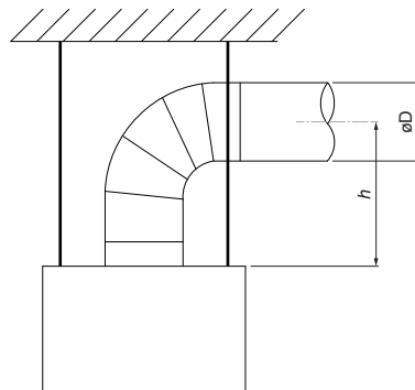
2. Freihängende Deckenmontage h_{\min} > (3 \sim 5) D
