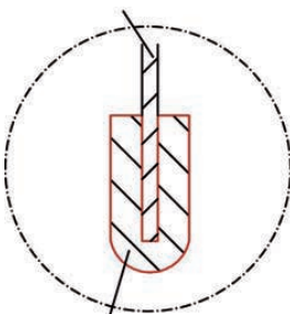
U-Dichtung lose
