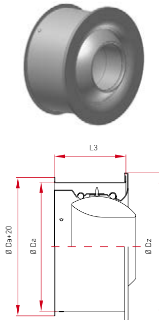
b) auf einem rechteckigen Kanal (K)
